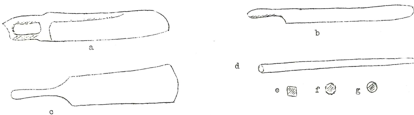
Fig. 7 a-c. Skäktsvärd. d. Skäktskäpp med e) fyrkantigt, f) åttasidigt och g) runt tvärsnitt.
