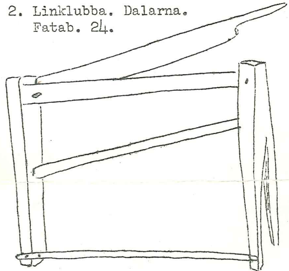
Fig. 3 b. Linbråka. Uppland. Fatab. 24.
